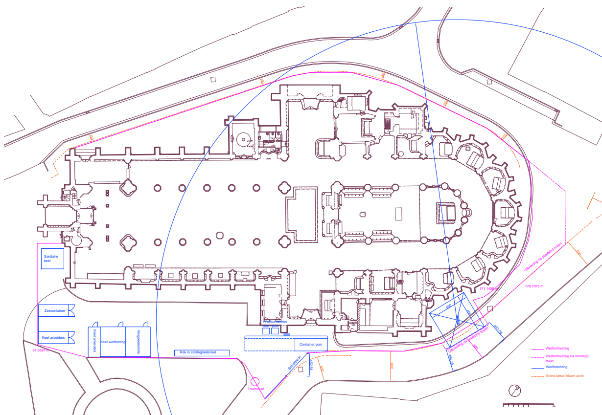
werfinrichtingsplan
